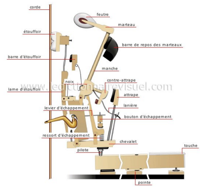
Le mécanisme du piano
