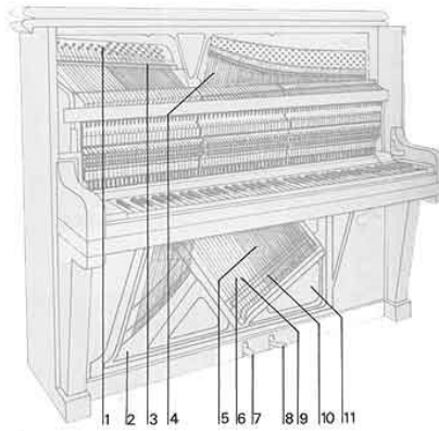
Le piano droit
