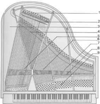
Le piano à queue
